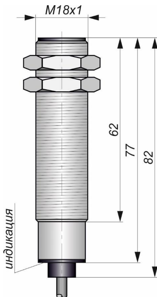
Габаритный чертеж
